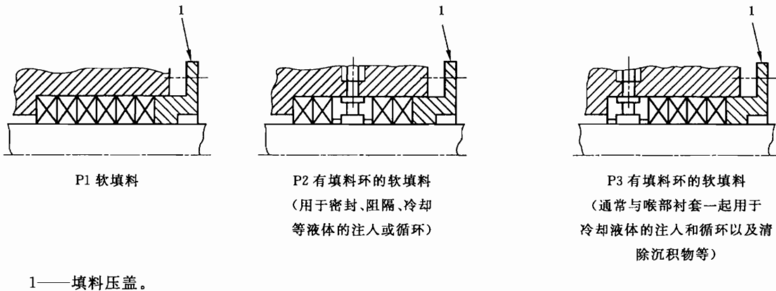
图 E.1 软填料密封的示例
